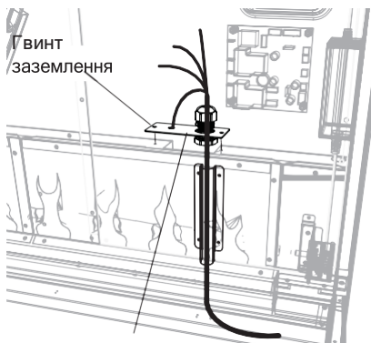
Кабельний затискач
